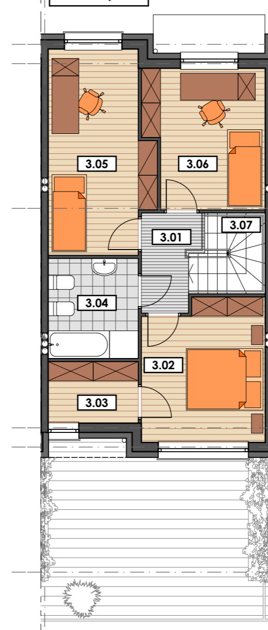
RZUT PIĘTRA
